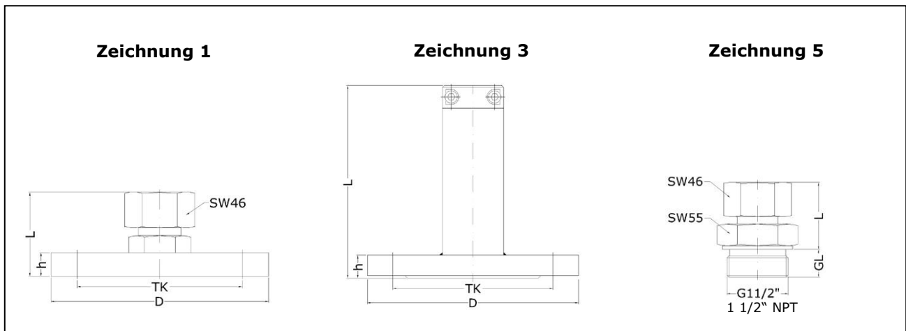
Sondenführungsteile SF
